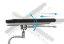
Armlehnensatz mit Linearführung und Einhandauslöser, ab-Werk-Montage
